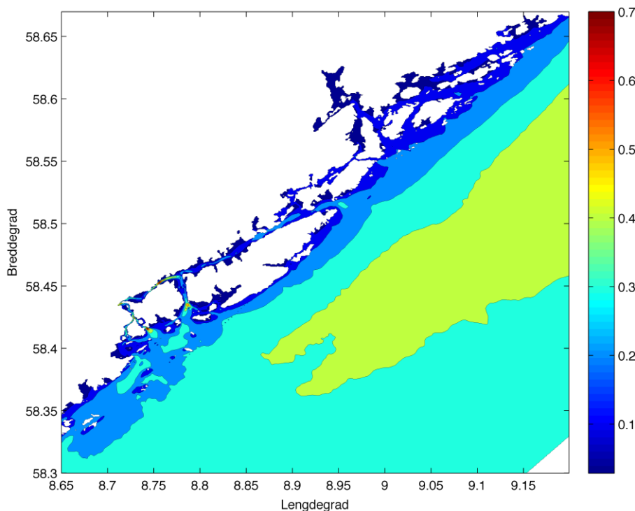
Figur 4. Modellert overflatestrøm midlet over en lengre tidsperiode. Fargeskalaen angir strømsstyrke i m/s. Retningen kommer ikke frem av dette kartet, men Kyststrømmen sin hovedretning er mot sørvest.
