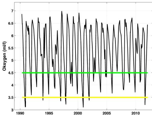
Figur 15. Variasjon i oksygen-forholdene i 140 m dyp (nær bunnen) i Ærøydypet de siste drøyt 20 årene. Forholdene svinger mye gjennom året fordi bunnvannet i Ærøydypet fornyes hvert år. Vannkvaliteten ut fra minimumskonsentrasjonene av oksygen i dypet ligger stort sett på God, det vil si mellom grønn og gul linje, men har enkelte år hvert mindre god (under gul linje), fra Kroglund m.fl. (2012).
