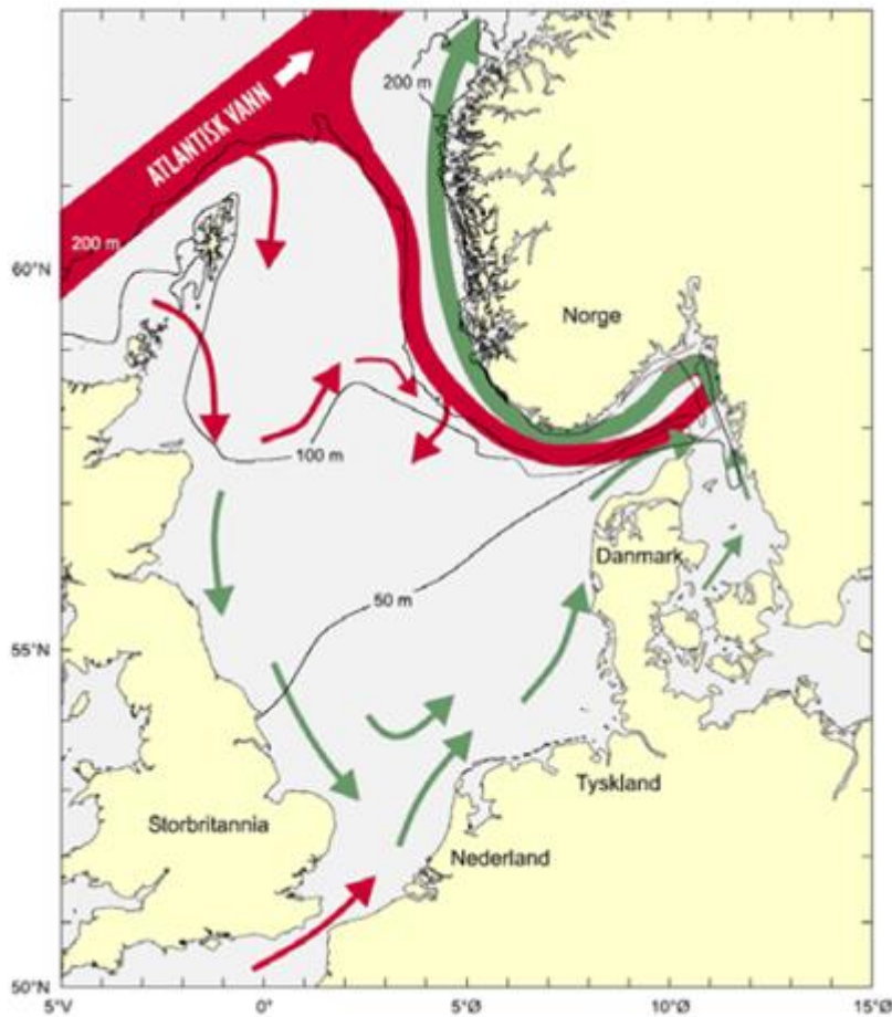
Figur 6. De generelle strømforhold i Skagerrak. Den norske kyststrømmen starter øst i Skagerrak og strømmer som en elv vestover (tykk grønn pil). Den er i store trekk lagdelt med atlantisk vann, som kommer inn fra vest, dypest (røde piler). Vann fra sentrale og sørlige del av Nordsjøen (Jyllandstrømmen, tynne grønne piler) ligger over det atlantiske vannet, og på toppen ligger et tynt lag med vann fra Østersjøen (også tynne grønne piler) sammen med tilførsler av ferskvann fra norske elver. Kyststrømmen setter særlig fart og går nær land ved østlige vinder, og bremses og presses ut fra land ved vestlige. Data: Havforskningsinstituttet.
