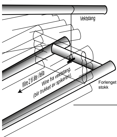
Fig 4. Utløsermekanisme (på fellas bakkant)
