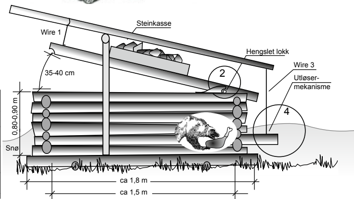
Fig 4. Utløsermekanisme (på fellas bakkant)
