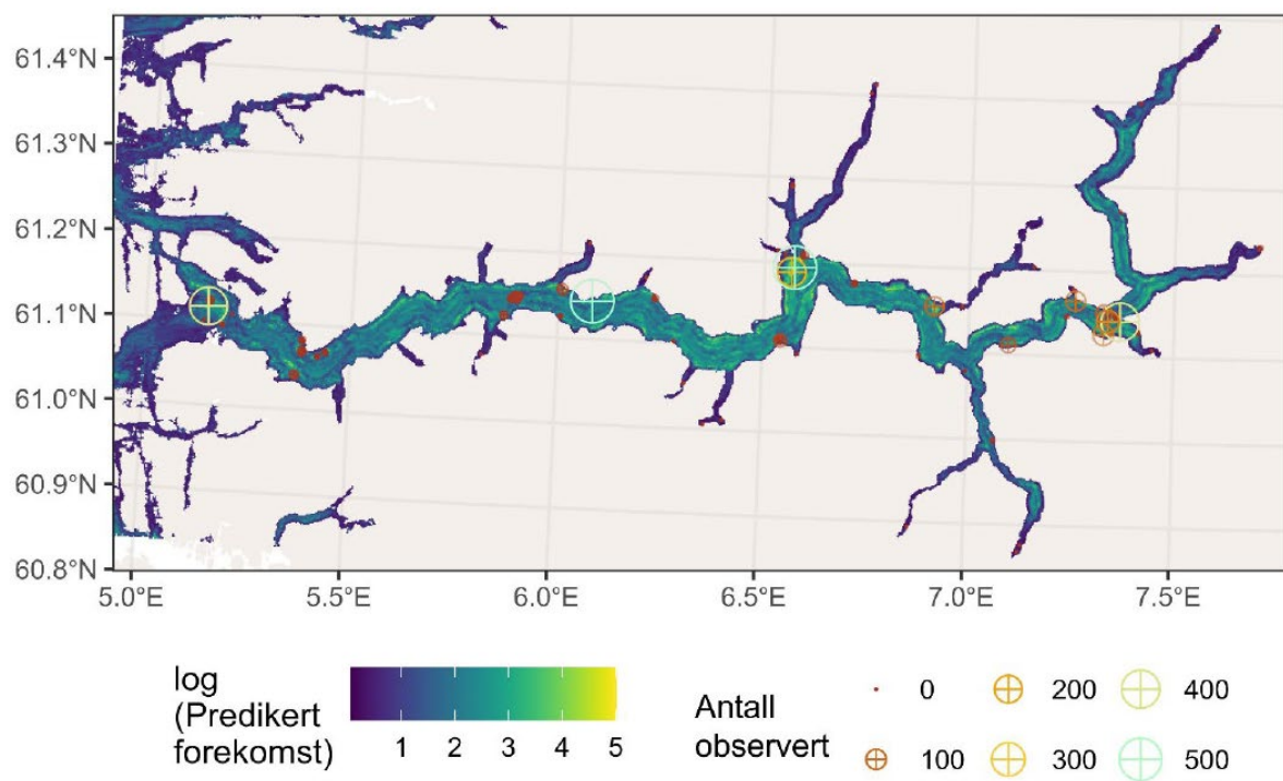
Figur 6.1-16 Modellert utbredelse av sylindersjørse bunn, hvor gul er høy sannsynlighet og blå er lav sannsynlighet. Observert sylindersjørse vises som sirkler. Figur fra Haugland m.fl. (2024).
