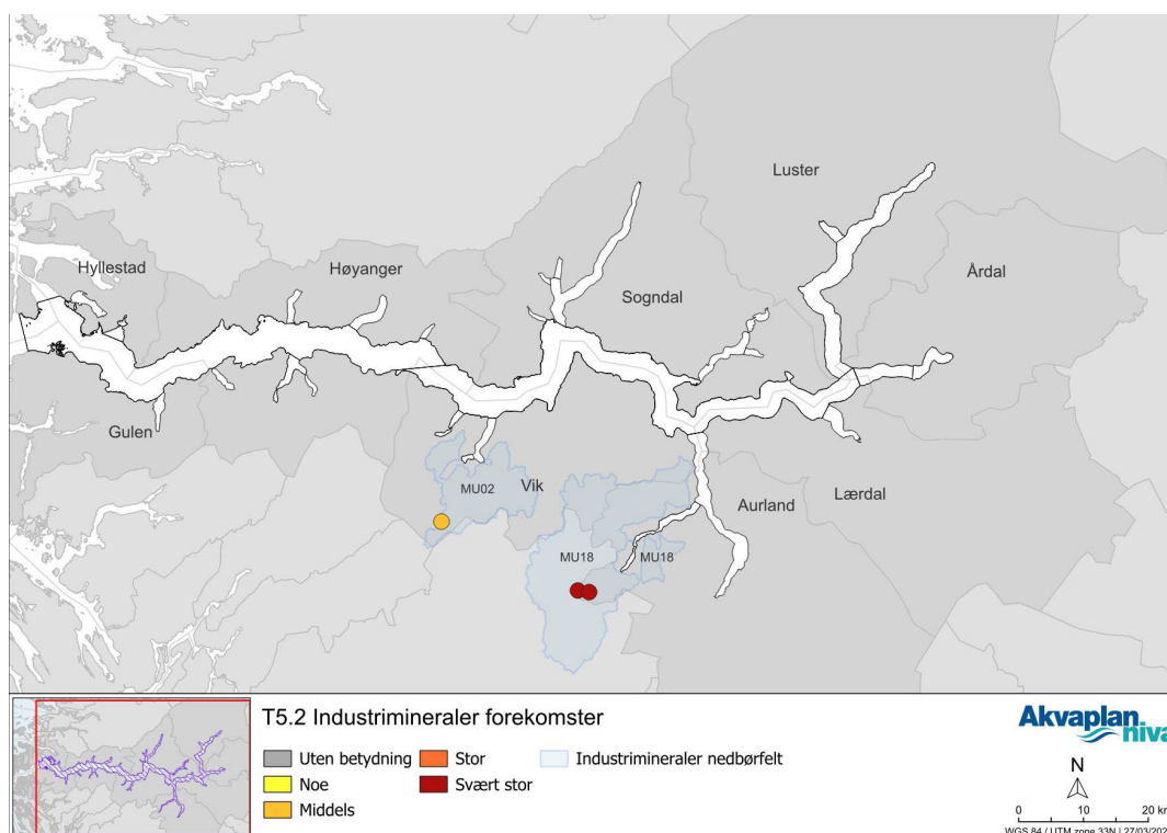
Figur 6.6-4 Verdisatte industrimineral forekomster. Nedbørsfelt som går ut i kandidatområdet merket med delområde kode som tilsvare delområdet nedbørsfeltet har utløp til (Datakilde: NGU/Mineralressurser).
