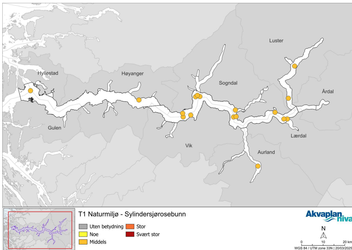
Figur 6.1-15 Registreringer av sylindersjørse bunn i Sognefjorden. Data fra Haugland m.fl. (2024) tilgjengelig på fylkesatlas.no.
