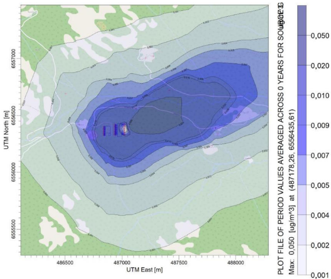
Figur 4-2: Årsmidlet bidrag av NO 2 , i µg/m 3 ved meteorologi for 2024. Nødscenario med 9 generatorer 2 timer.
