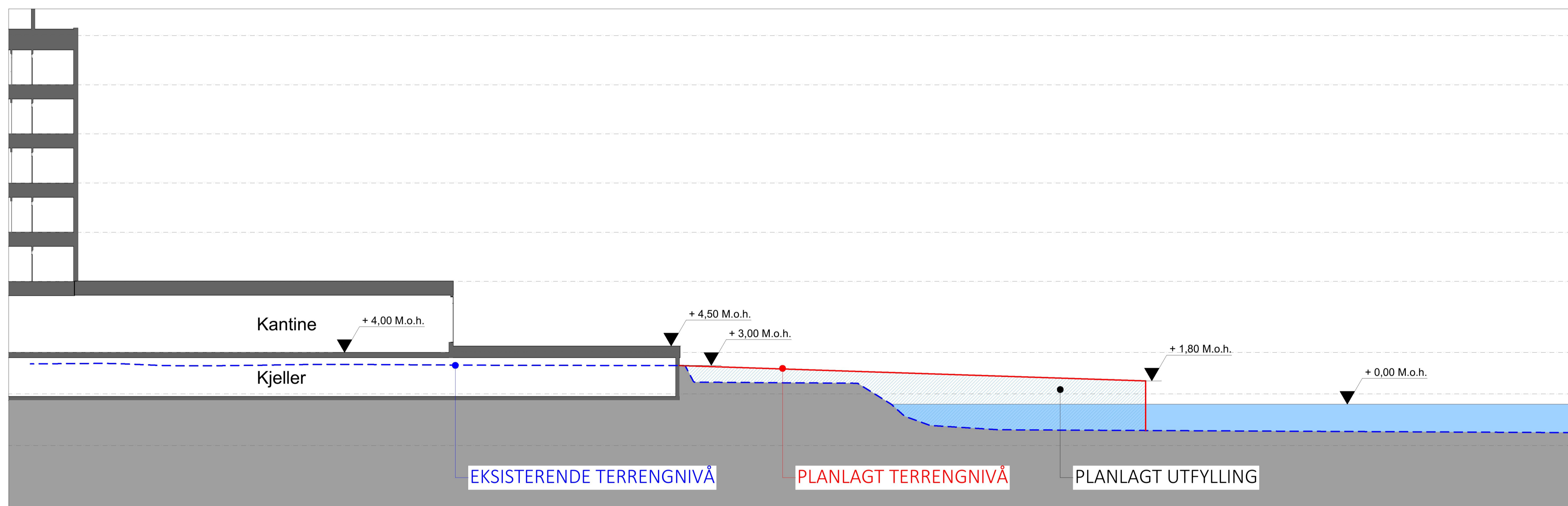
Snitt Kantine
