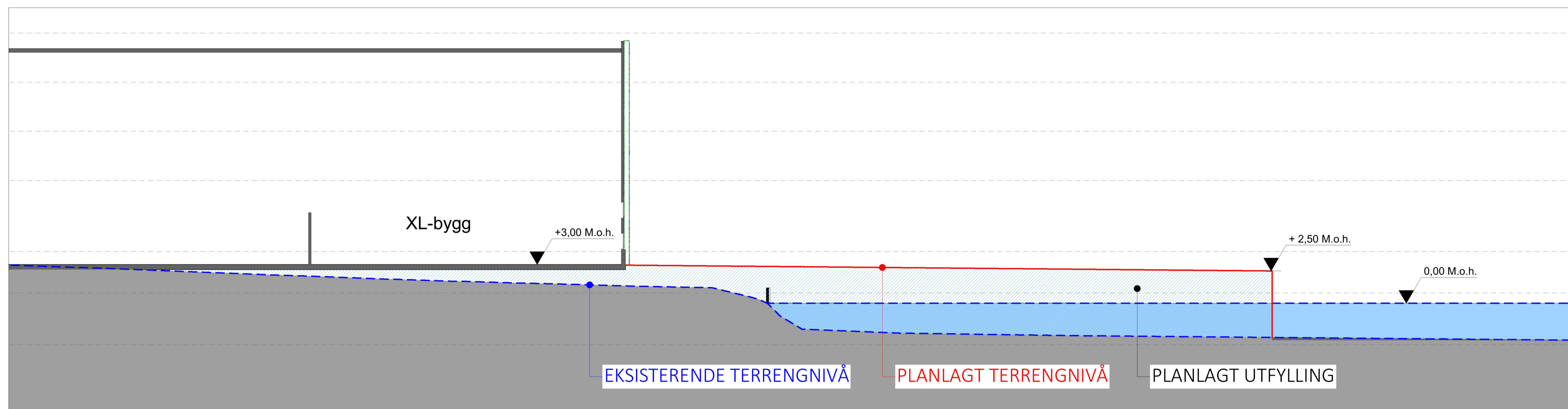
Snitt XL-bygg
