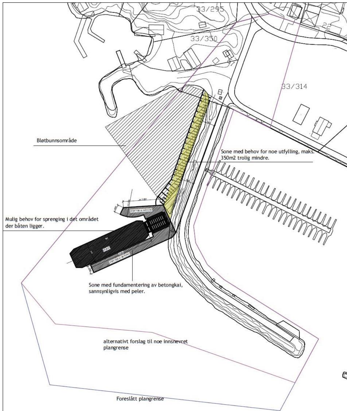
Figur 2. Planskisse av det nye fergeleiet på Sandøya. Merk at ferga er tegnet inn i illustrasjonen.
