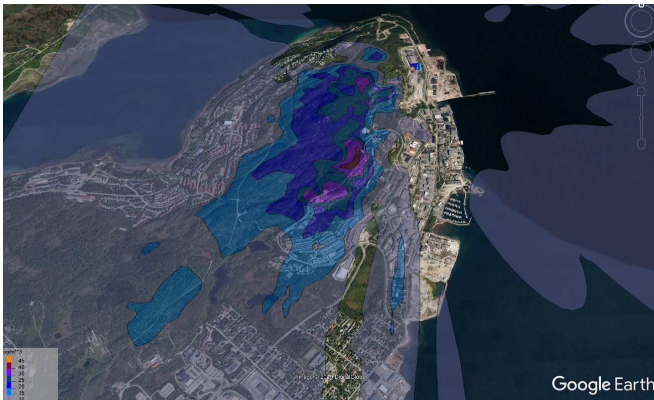
Figur 3 Maksimalt timemidlet bidrag av NO 2 ( \mu\text{g}/\text{m}^3 ) ved utslippskonsentrasjon 200 \text{ mg}/\text{Nm}^3 \text{ NO}_x . Skorsteinshøyde på 60 meter på eksisterende linjer og ny linje
