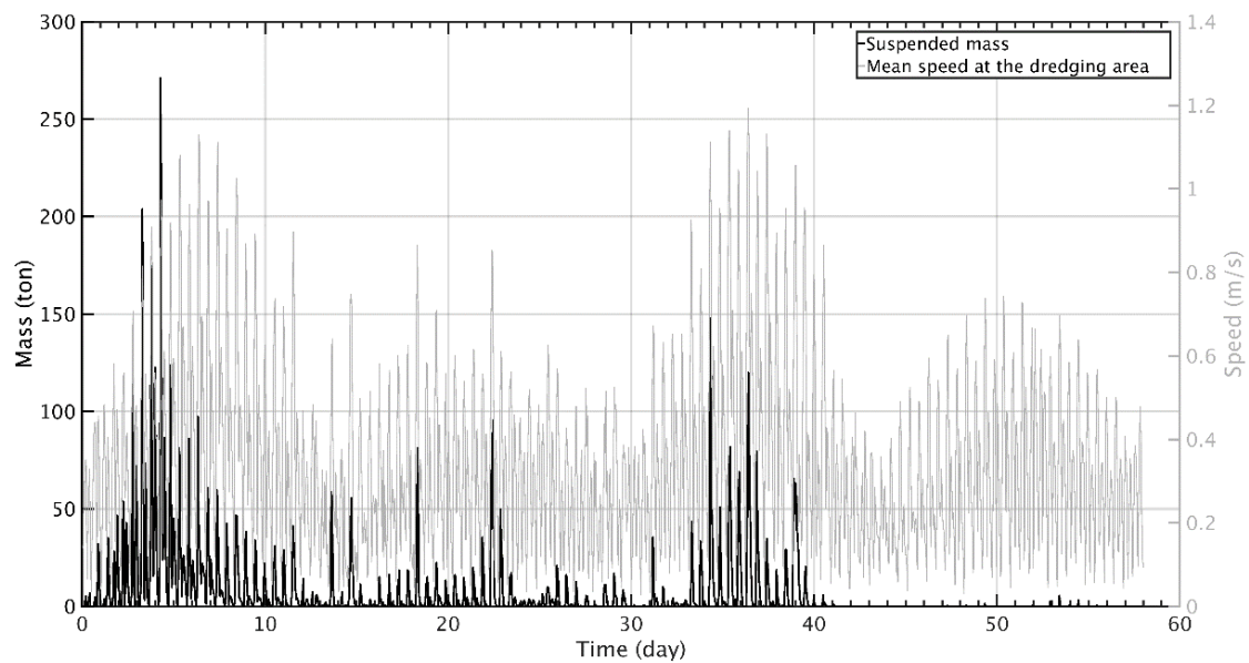
Figur 10. Tidsserie av mengden suspendert masse i vannsøylen (sort kurve) for grabbmudring (øverst) og sugemudring (nederst). Strømstyrken i mudringsområdet (gjennomsnitt fra de to mudringsområdene) er vist med grått
