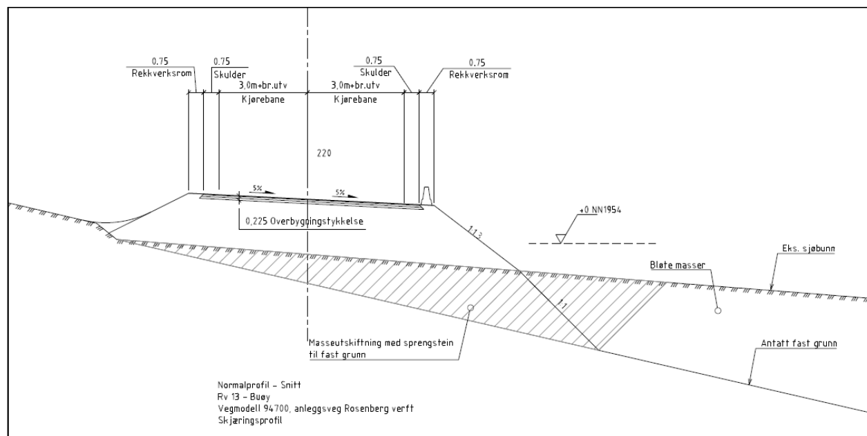
Figur 3 Masseutskifting snitt
