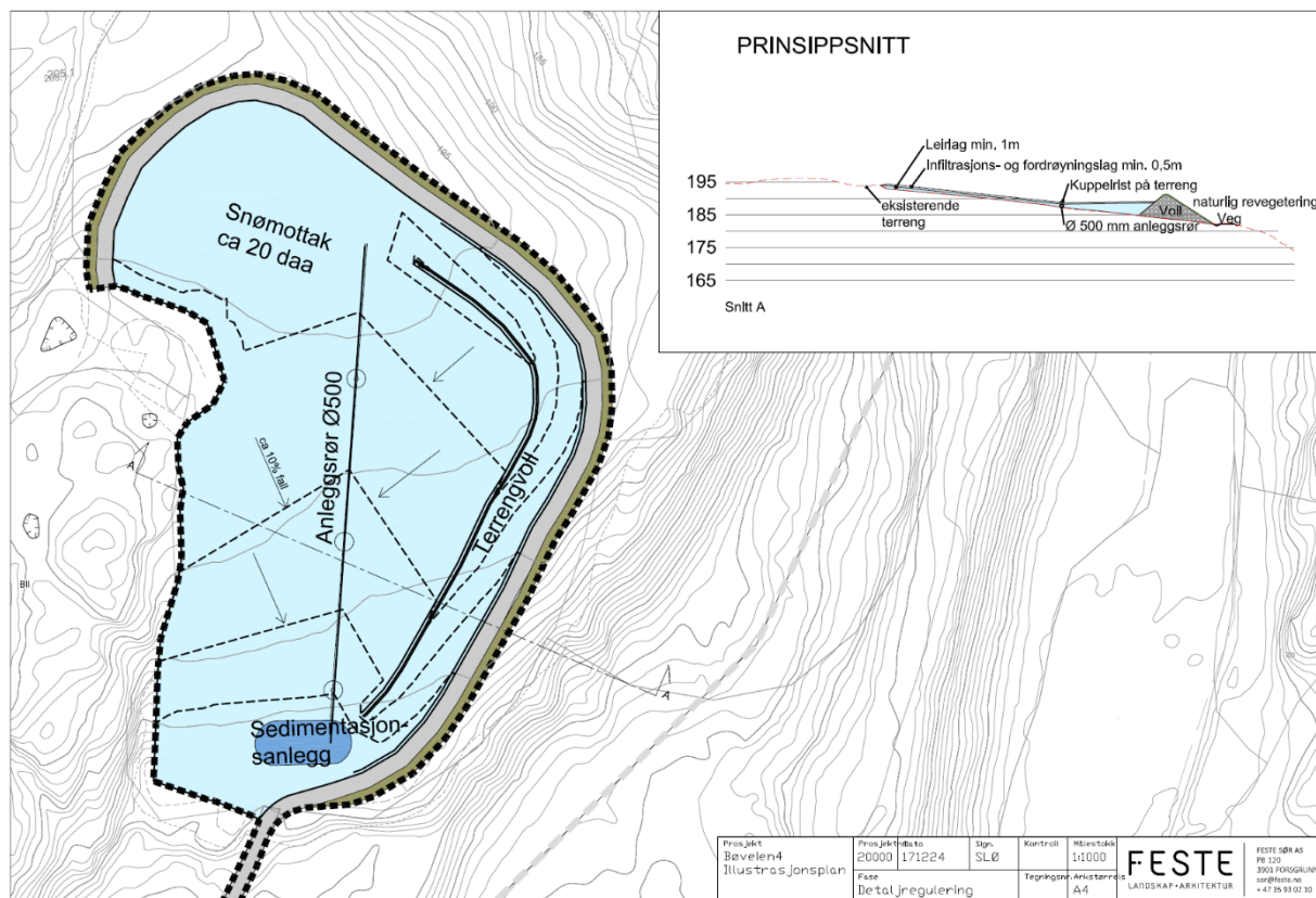
Figur 1: Illustrasjonsplan med snitt - prinsippsskisse for utforming
