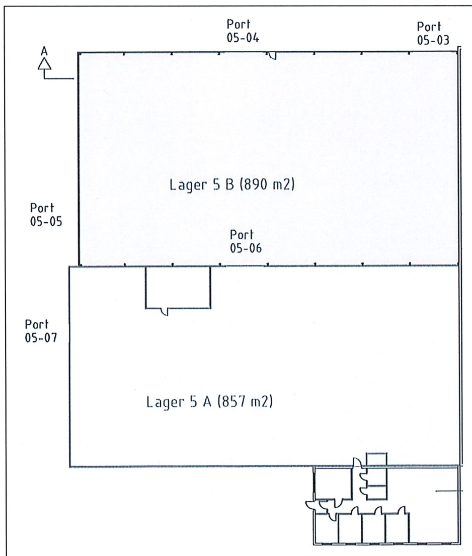
Havnelager 5 oversiktstegning
