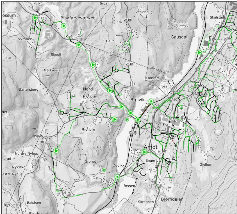
Figur 21. Kartutsnitt av ledningsnett og pumpestasjoner innenfor Bårud avløpsanlegg. Grønne linjer indikerer spillvannsnettet, og sorte linjer overvannsledninger.
