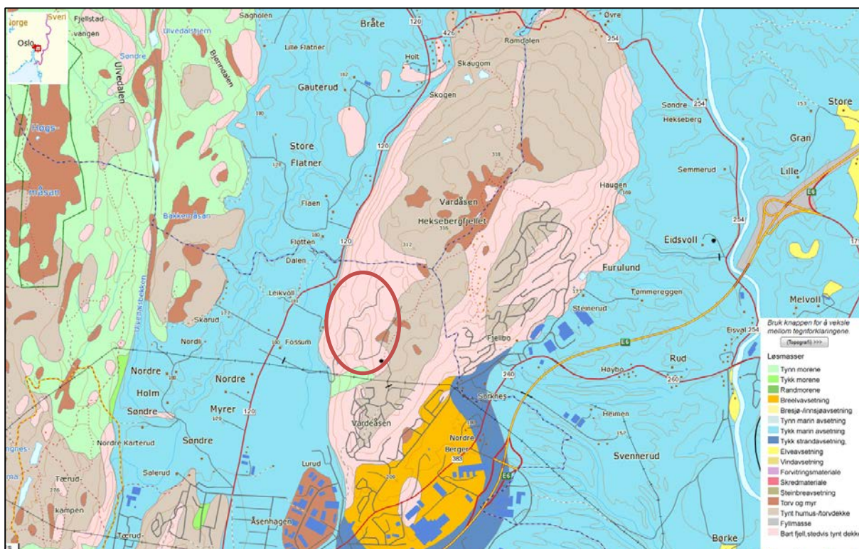
Figur 3 Løsmassekart fra NGU (rød sirkel viser steinbruddets lokalisering)
