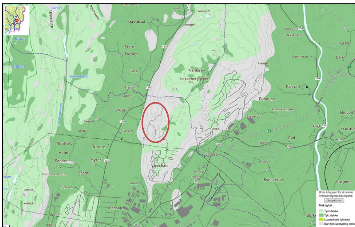
Figur 4 Kart med jordmassenes mektighet (rød sirkel viser steinbruddets lokalisering)
