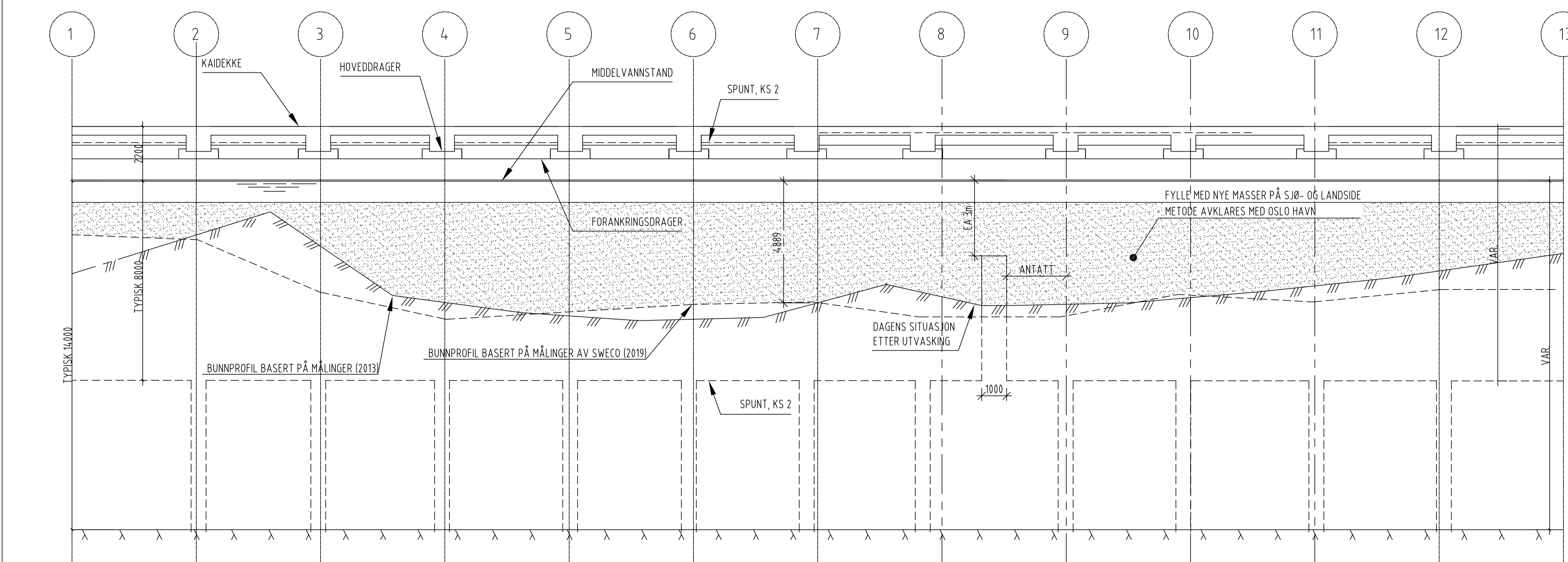
SNITT 1 - 1 1:100
