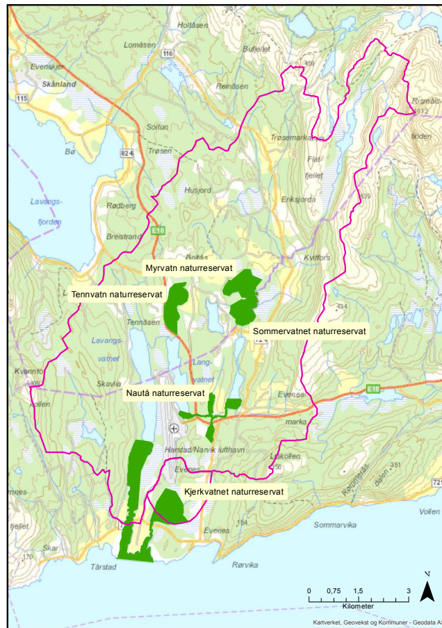
Figur 2: Tårstadvassdraget nedbørfelt og delteft Kjerkvatnet med utløp mot Ofotfjorden. Kilde NVE og Holtan & Brettum 1995
