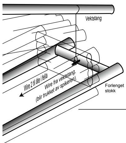
Fig 4. Utløsermekanisme (på felleas bakkant)
