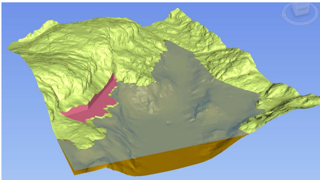
Figur 4. 3D-modell av området som viser terrenget over og under vann. Området som skal sprenges ut er lagt inn i modellen (rødt område). (Modell: Multiconsult)
