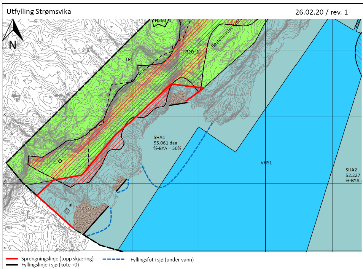
Figur 3. Utsnitt av detaljreguleringsplan (Cowi). Planlagt fjellskjæring etter sprengning er vist med rød linje. Brun tekstur viser fyllingsarealet over vann og blå, stiplet linje viser antatt fyllingsfront på sjøbunnen.
