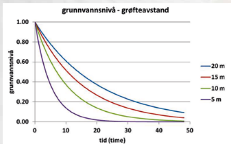
Figur 1: Viser sammenheng mellom grunnvannsnivå (1,0 er jordoverflata) og tid det tar å senke grunnvannsnivået ved ulike grøfteavstand. Illustrasjonen er fra ei jord med god mettet vannledningsevne.
