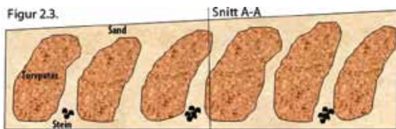
Figur 2, teikna av Nono Dimby.. Omgraving med tverrstilte skrålag trinn for trinn. Figur 2.3. er eit snitt vinkelrett på arbeidsgrøfta etter at den er fyllt med torvputer og sand. Linja, snitt A-A, markerer planet figur 2.2. ligg i. Som ein ser i figur 2.3 er sandfeltet laga i trinn 4 i figur 2.2. samanhengande frå overflata og ned i undergrunnen. Mellom arbeidsgrøftene er det kompakt torv under 40 – 50 cm sand.
