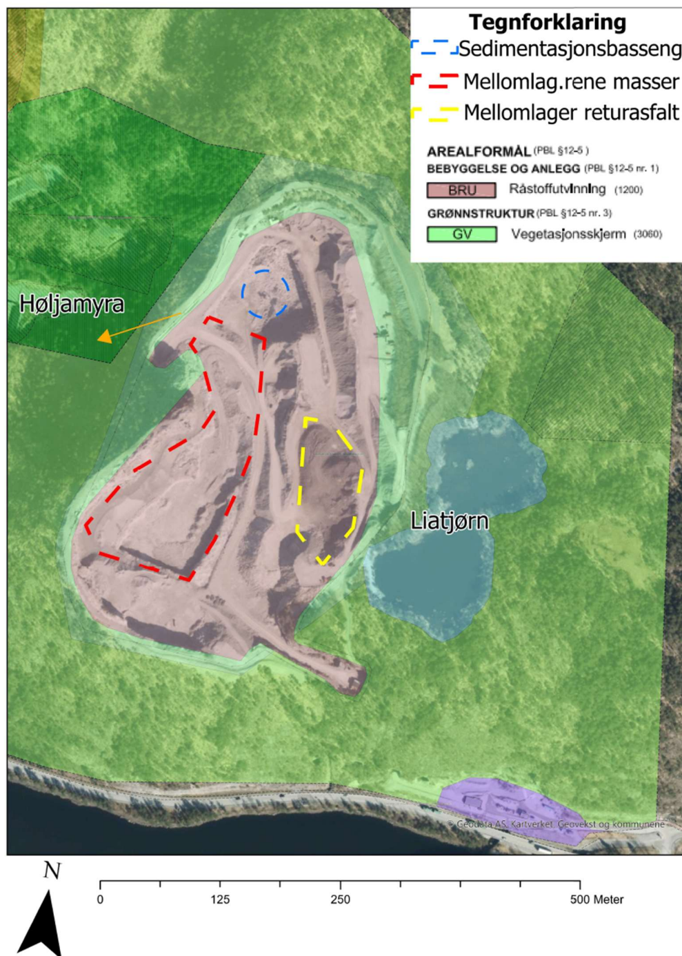
Figur 4-3: Kartutsnittet viser planlagt plassering av mellomlager for rene masser i dagbruddet, innenfor rød, stiplet linje. Gul stiplet linje viser plassering av mellomlager for returasfalt, mens blå stiplet linje viser lokalisering av sedimentasjonsbasseng. Farget bakgrunn indikerer også arealformål etter gjeldende reguleringsplan. Kartkilde: ArcGIS.
