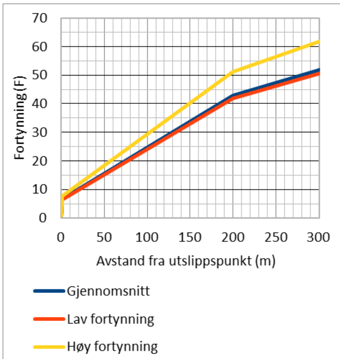
Figur 15. Utslipp i overflaten til kystvann. Figuren viser estimert fortynning ( F = antall ganger) i økende avstand fra utslippspunkt (m). Kilde: Miljødirektoratet - faktaark M-1288:2019 [31].
