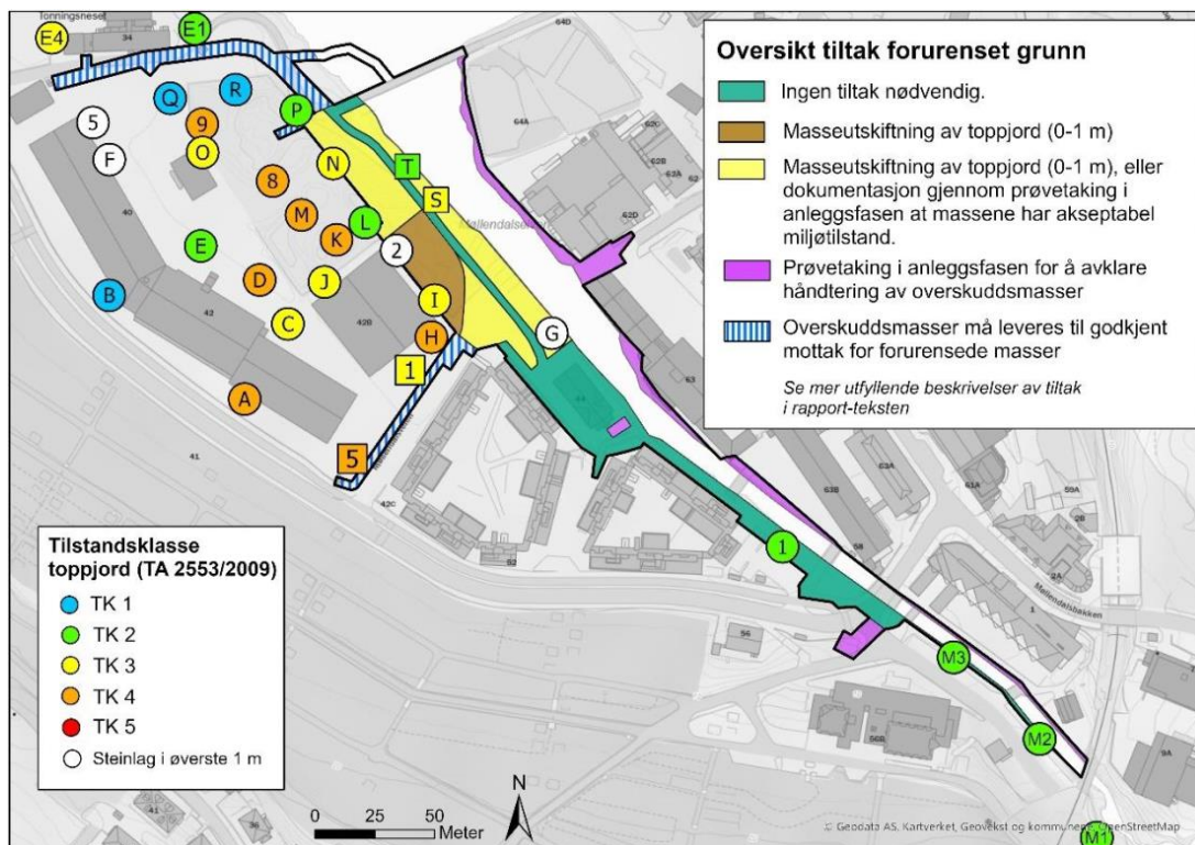
Figur 4 Oversikt over anbefalte tiltak mot forurenset grunn. Tilstandsklasser for jordprøver er i henhold til klassifiseringssystem gitt i TA 2553/2009. Sirkler viser jordprøver tatt med borerigg, og firkanter viser jordprøver tatt med gravemaskin.
