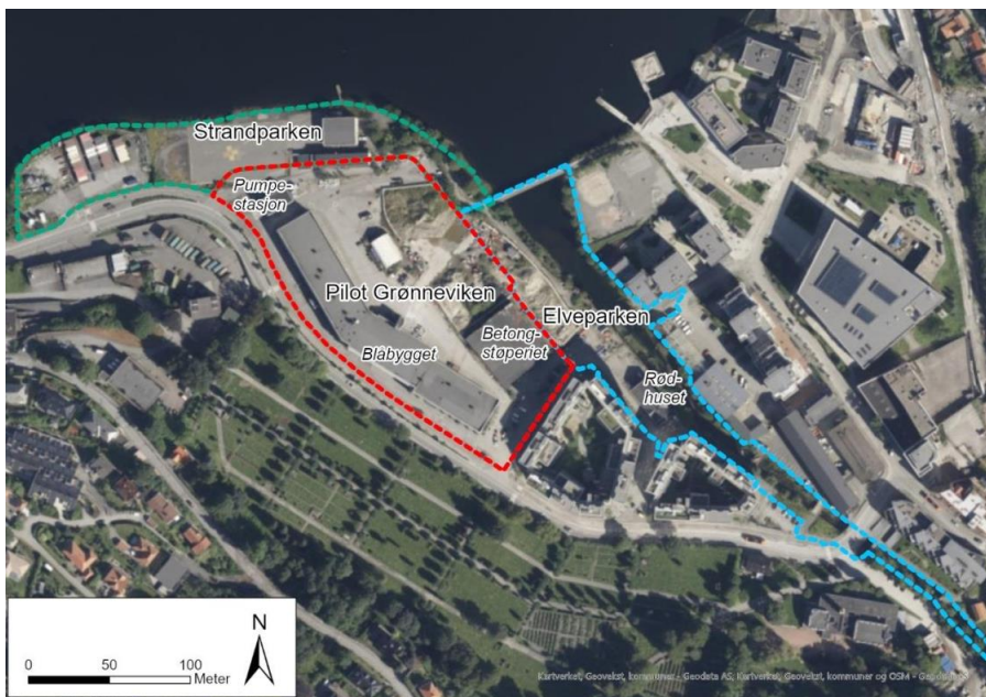
Figur 1 Flyfoto over området som viser de tre prosjektområdene Pilot Grønnevik, Elveparken og Strandparken med dagens bygningsmasse.
