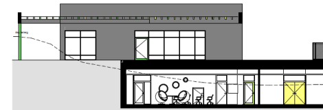
Vest - Hovedinngang
