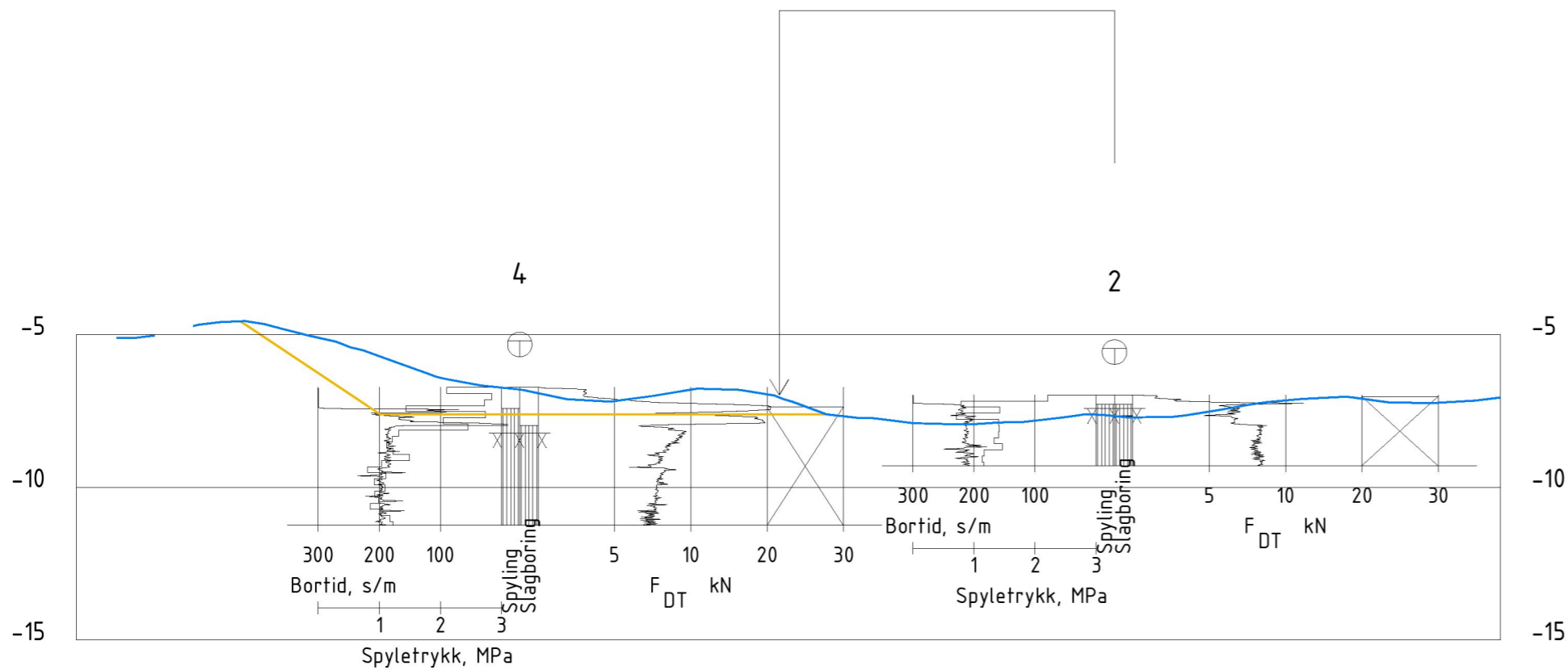
Profil B-B
