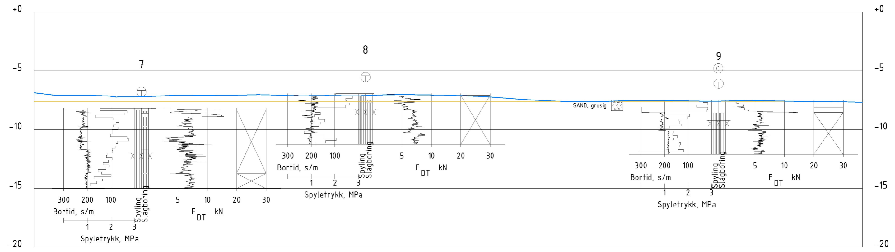
Profil E-E
