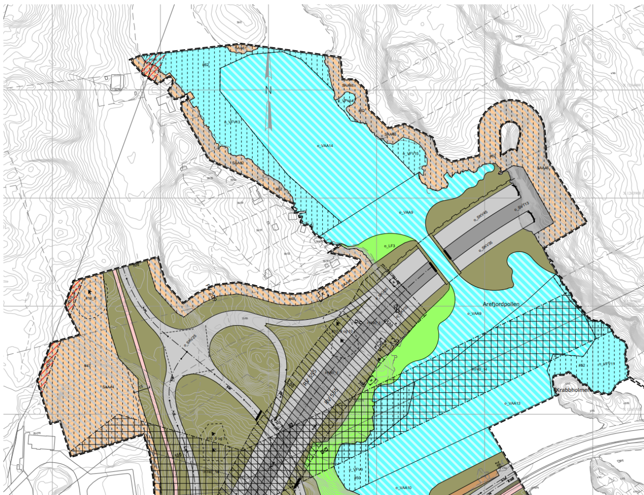
Figur 4 - Plantegning av kulvert/voll ved nordre del av Arefjordpollen. Hentet fra plankart 11.1, Fjell kommune parsell 3 [8].
