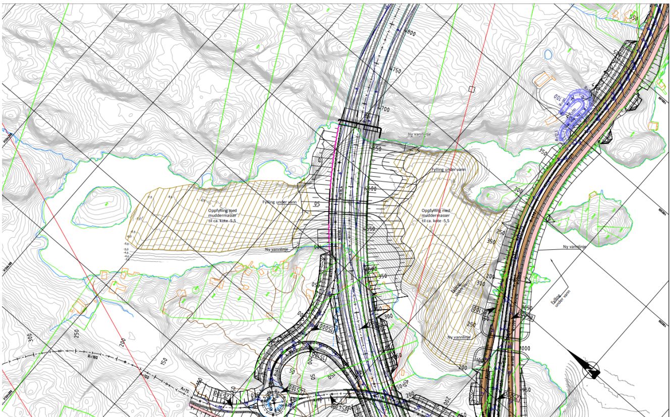
Figur 10 - Oppfylling med muddermasser til ca. kote -5,5 er vist med brun skravering på begge sider av vegfylling i tegning D138.Reguleringsplantegninger.
