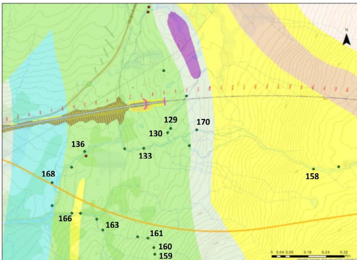
Figur 11. Nummerering og plassering av berggrunnsprøver fra vestre siden av Kvænangsfjellet.
