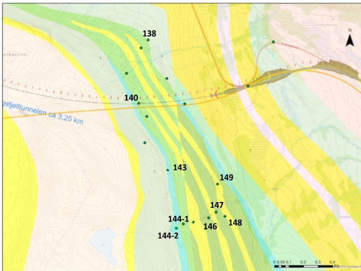
Figur 10. Nummerering og plassering av berggrunnsprøver fra østre siden av Kvænangsfjellet.
