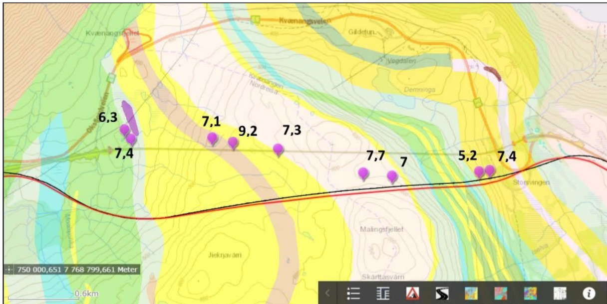
Figur 12. Feltnmålinger av pH i bekker og tjern langs en tidligere foreslått veitrase gjennom Kvænangsfjellet. Det er målt noe lavere pH i og nedstrøms områder preget av skifer. Vegetasjonen i områder med skifrig berggrunn er dominert av myr, noe som forventes å senke pHen i vannfasen.
