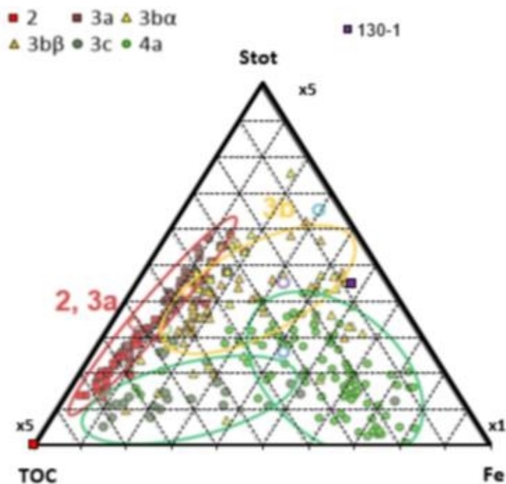
Figur 9. Trekantendiagrammet viser at prøve 130-1 (lilla firkant) har lavt innhold av TOC i forhold til svovel og jern, og plotter nær etasje 3bβ. Skifre med størst syredannende potensiale plotter i etasje 2 og 3a.
