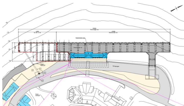
Figur 1 Oversiktstegning kaiutvidelse
