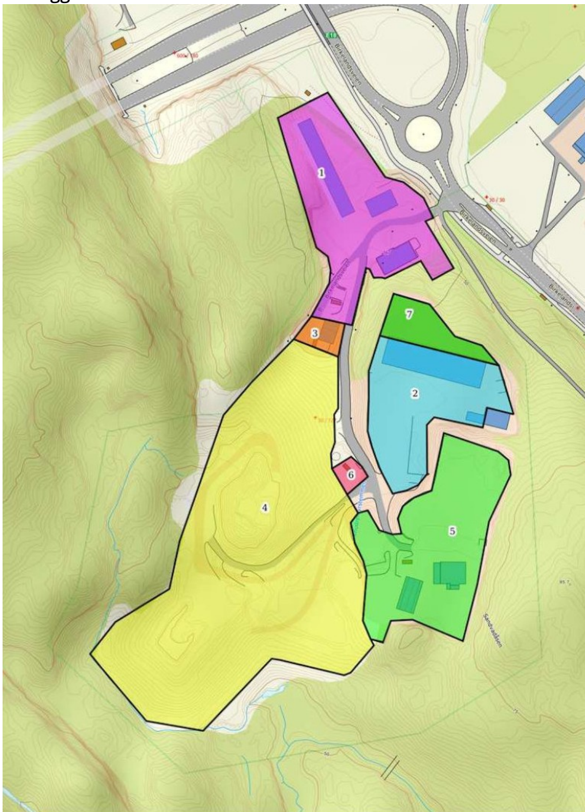
Bilde 1: Oversiktsbilde med beskrivelse av ulike aktiviteter og overvannshåndtering på anlegget. Forklaring for områder: 1 = gjenvinningsstasjon, 2 = sorteringsområde, 3 = prøvetakingsområde, 4 = deponi, 5 = lager og parkeringsområde, 6 = vaskeplass, 7 = lagerområde for tomme containere.
