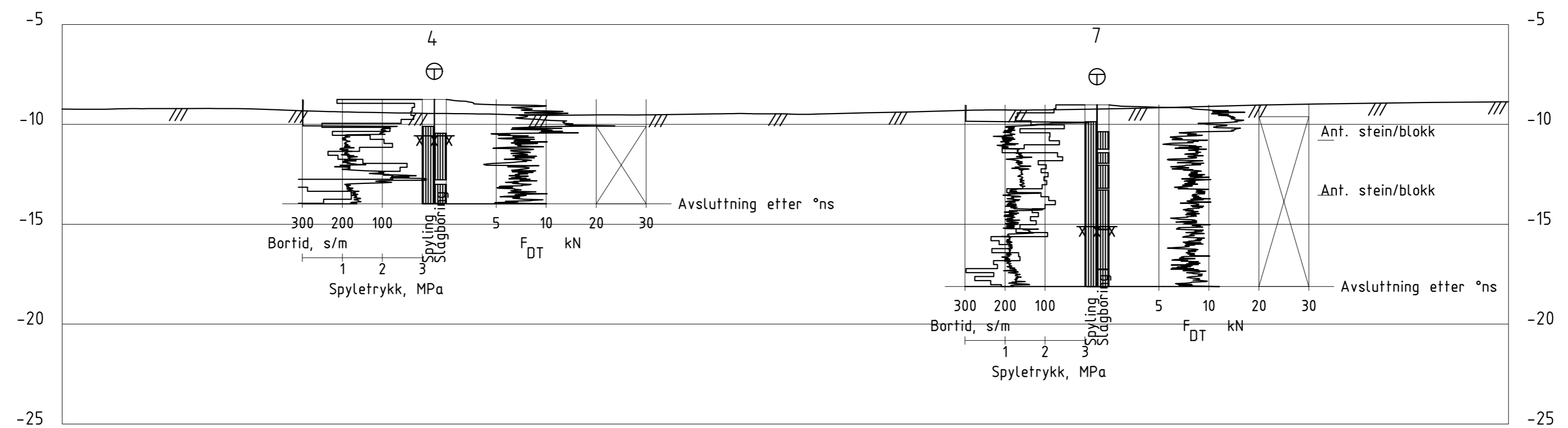
Profil B-B 1 : 200
