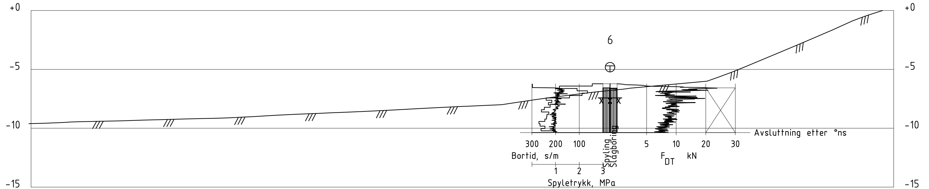
Profil D-D 1 : 200
