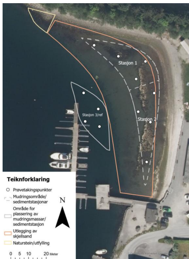
Figur 3: Sedimentstasjonar ved mudring- og dumpingområdet i Etne.
