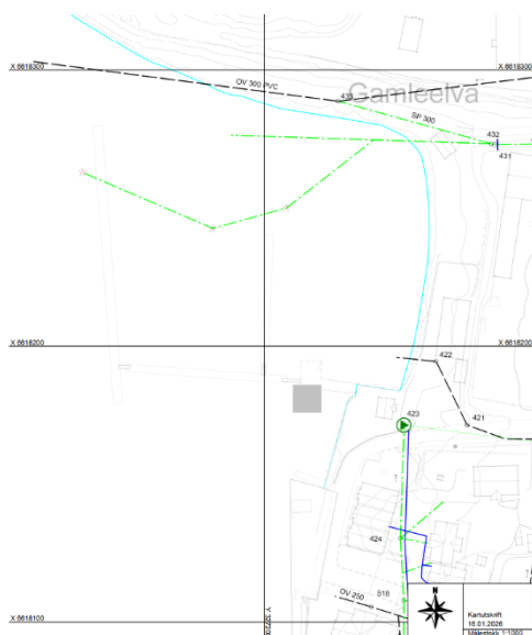
Figur 4: Eksisterande og planlagde leidningar ved Etne båthamn.
