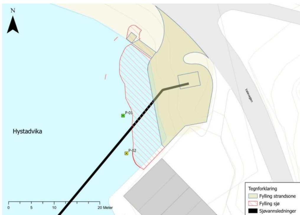
Figur 2 Utsnitt av tegning som viser planlagt utfylling og plassering av ledning i Hystadvika, samt plassering av prøvetakingsstasjonene P-01 og P-02 i tiltaksområdet for utfylling.
