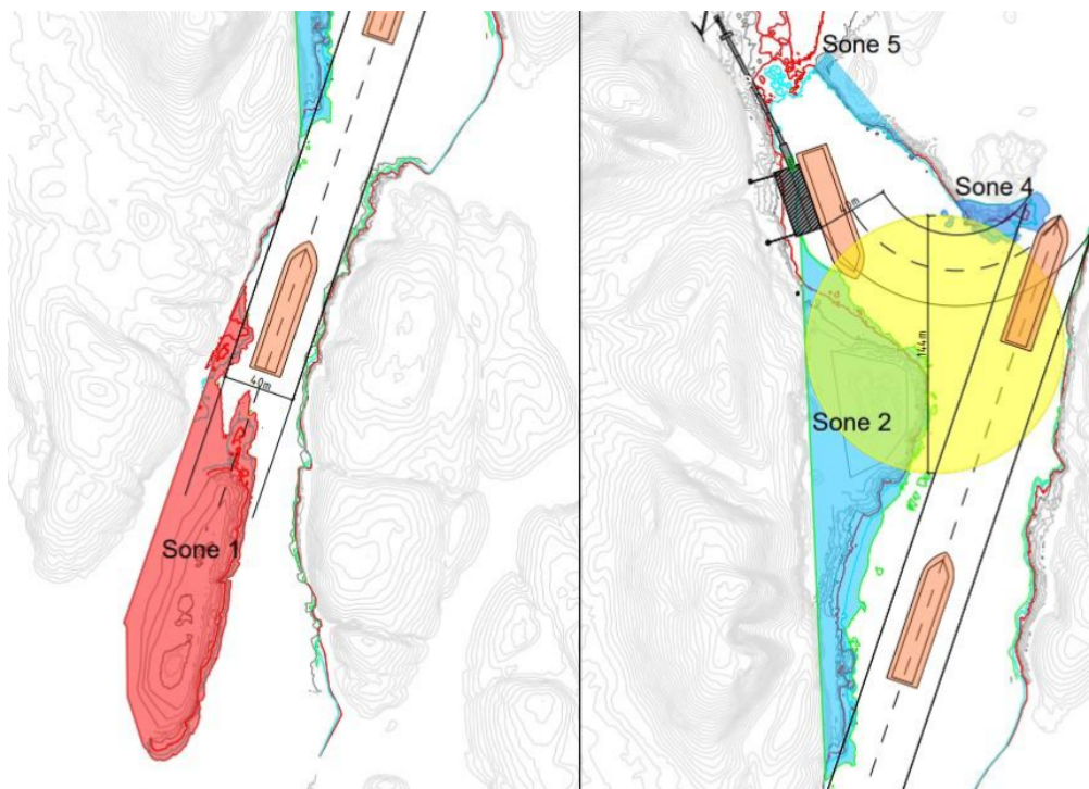
Figur 1: Situasjonsplan for mudrings- og undervasssprengingsområdet i Langøysundet. Hentet frå «Søknad om dispensasjon for utbetring av farlei i Bulandet – Askvoll kommune».
