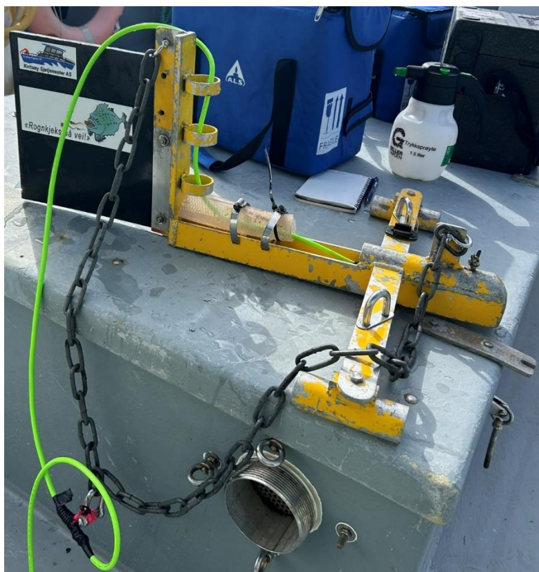
Figur 2-1 Installasjon for dropkamera laget av Kvitsøy Sjøtjenester AS. Dropkamera er festet inne i metallrammen og senkes ned med kabel. Styrefinne på metallrammen gjør at det er enklere å styre dropkameraet under fremdrift med båt.
