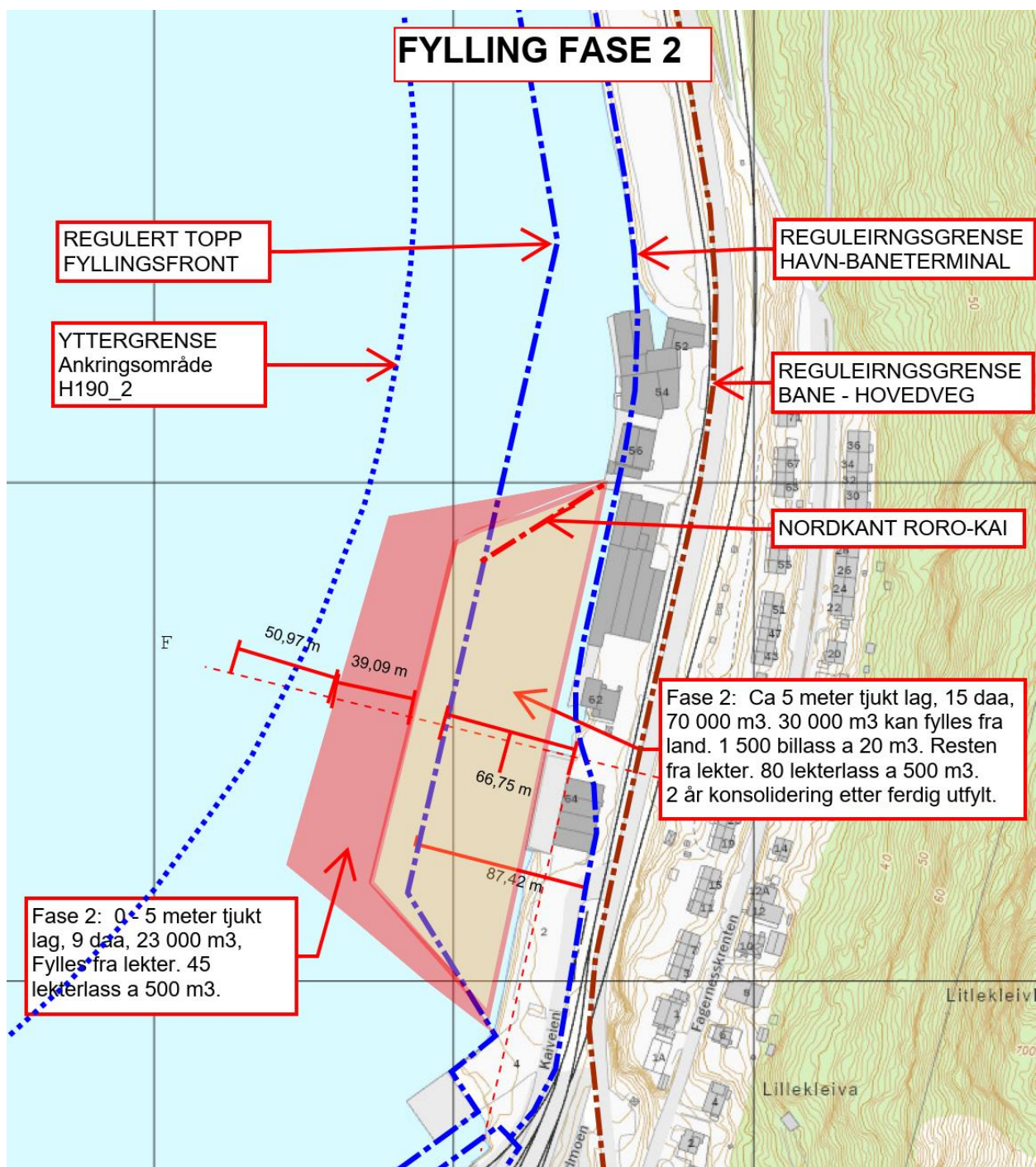
Figur 14 Roro-fylling, fase 2
