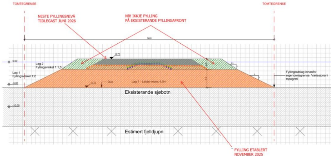
Figur 1 Tverrsnitt utfylling som viser etappe 2
