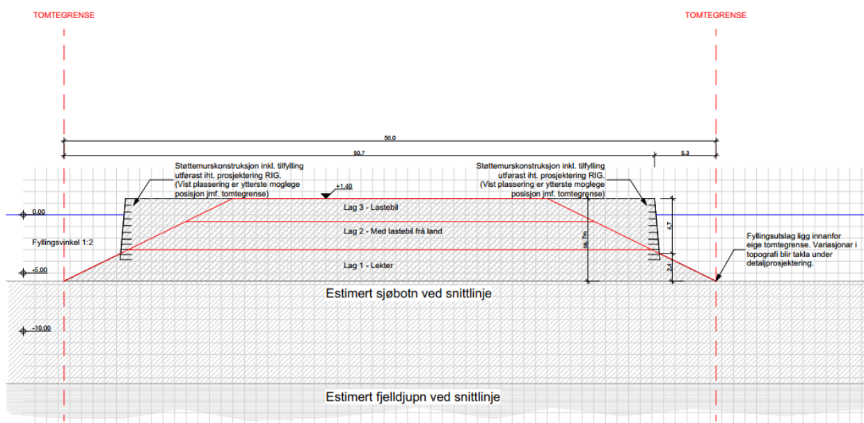
Figur 3: Terrangsnitt med prinsipp for fyllingsfot i sjø mot tomtegrense.
