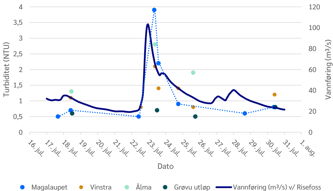
Figur 19. Turbiditet ved stasjonene Mågålaupet, Ålma, Vinstra og Grøvu utløp under første behandlingsperiode. Vannføringen ved Rise er hentet fra Sildre.no (stasjon 109.9.0).
