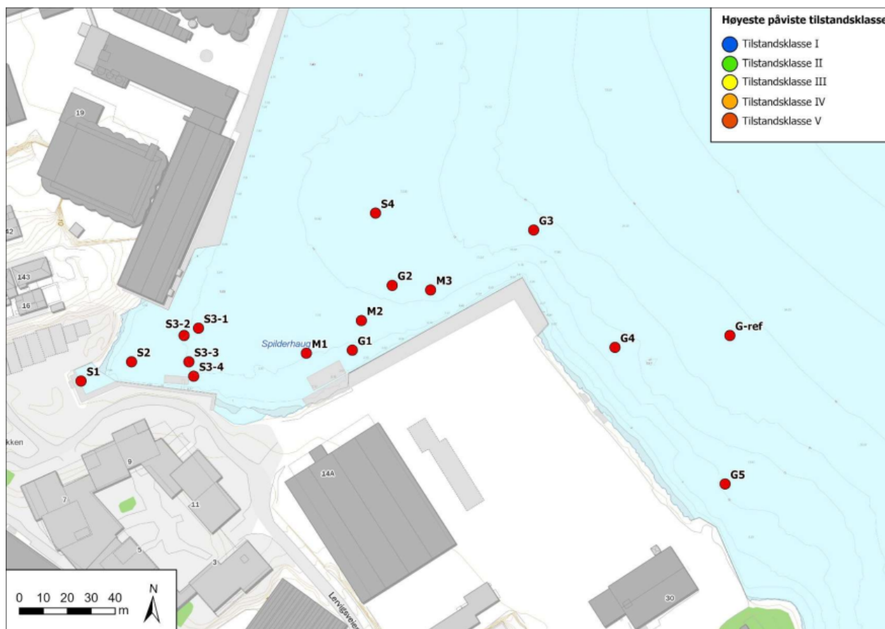
Figur 2 - Oversiktskart over tiltaksområdet med prøvetakningsstasjoner klassifisert med fargekoder for tilstandsklasser iht. gjeldende veileder M-608. TBT (tributyltinn) er klassifisert ved bruk av forvaltningsmessig tilstandsklasse. Figuren er hentet fra søknad og Norconsult Norge AS sin miljøtekniske sedimentundersøkelse.
