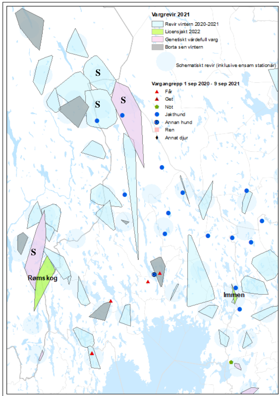
Figur 2. Underlag för urval av revir enligt kriterier. Kartan visar vargangrepp från och med 1 september 2020 till 9 september 2021 samt om det finns genetiskt värdefulla individer i reviren. Kartan ger även en bild av var tätheten är som störst och därmed får störst påverkan på älgförvaltningen. Revir där det finns vargar med fungerande sändare har markerats med "S". Revir där en eller båda vargarna revirmarkerande paret har försvunnit sedan vintern 2020-2021 har inte tagits med i urvalet för revir. Detta gäller reviren Stora Bör, där licensjakt genomfördes 2021, Skugghöjden, där hanen avlivades av djurskyddsskäl pga hög ålder och skada, samt Skacksjöreviret där hanen avlivades med stöd av 28 § jaktförordningen under sommaren 2021.
