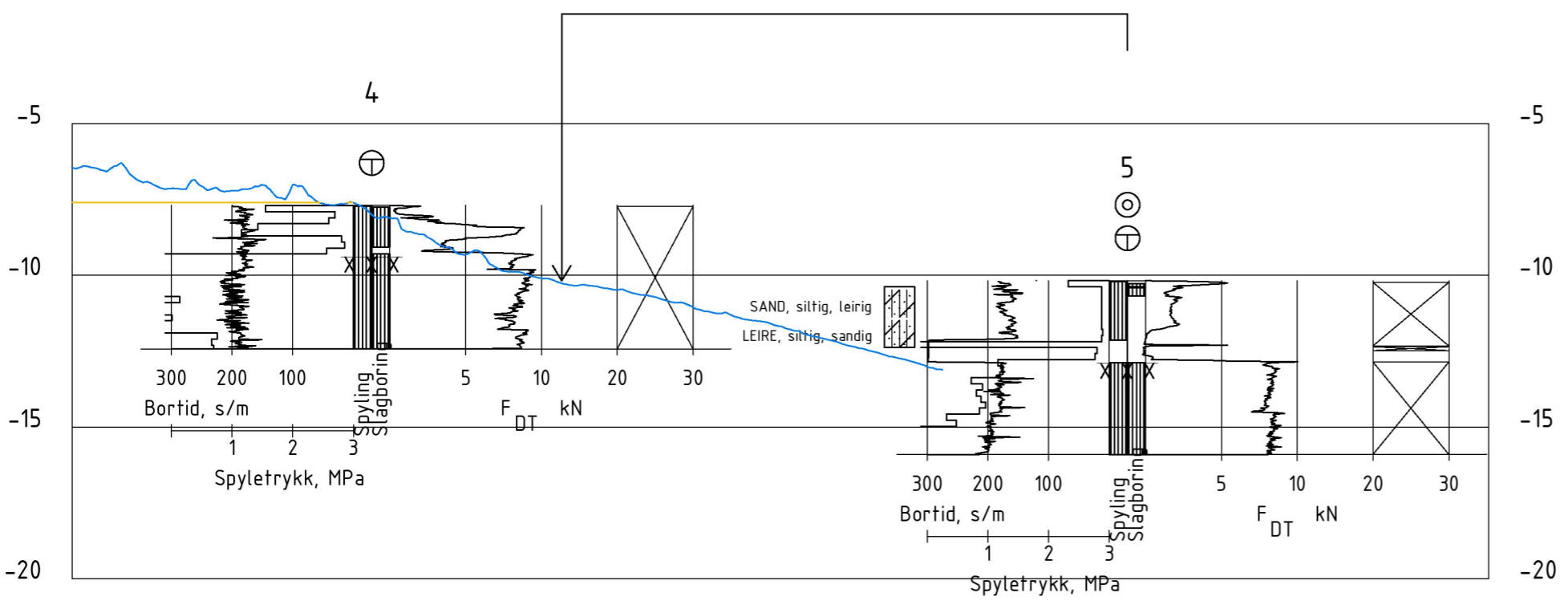
Profil B-B
