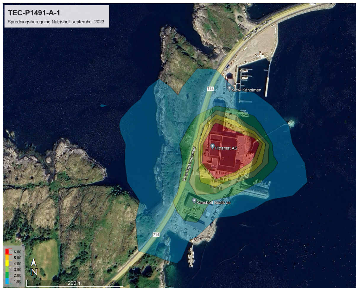
Figur 3.3: Modellering av lukt for Nutrishell Hitra. Maksimal månedlig 99 prosent timefraktil. Plottet 1-6 \text{ou}_E/\text{m}^3 .
