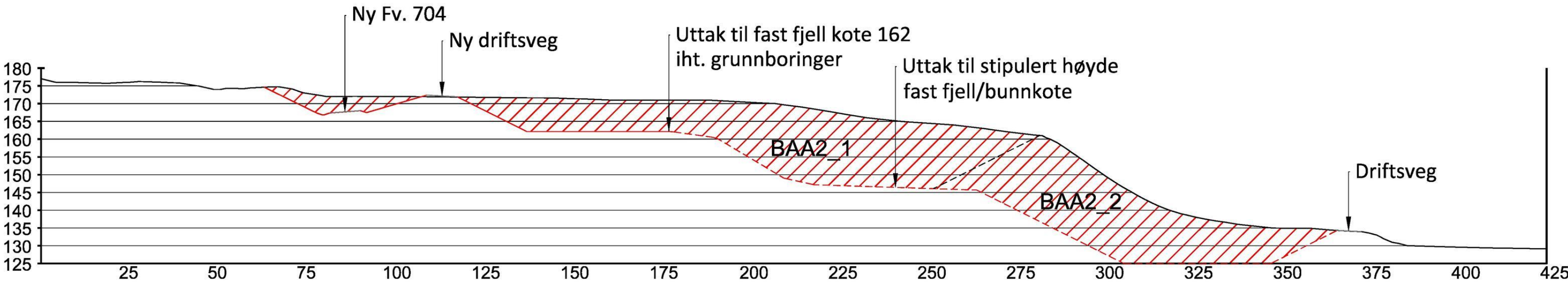
Snitt B - B'
