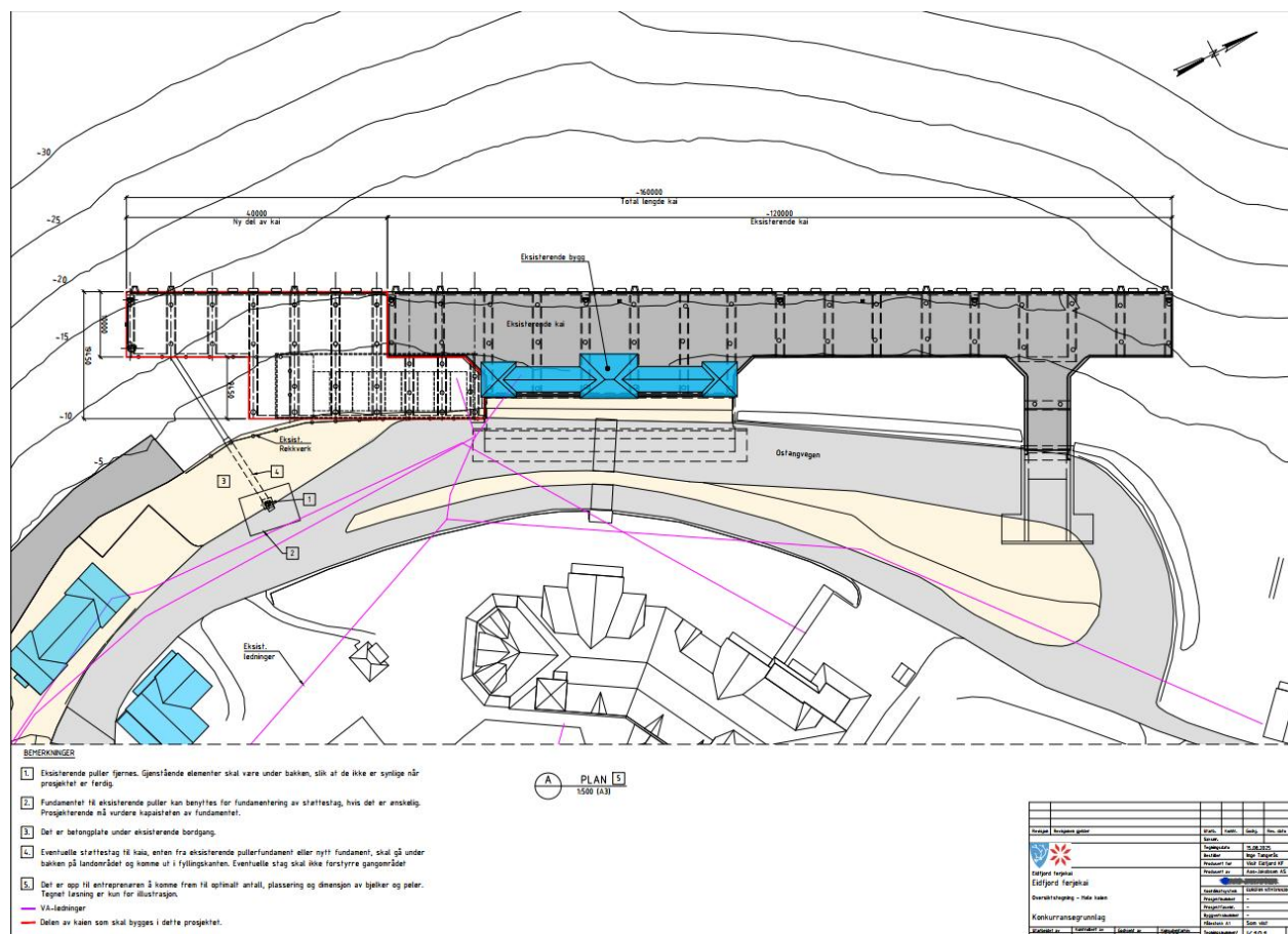
Figur 2: Tegning over planlagt arbeid. Rødt omriss viser delen av kaien som skal bygges i dette prosjektet.
