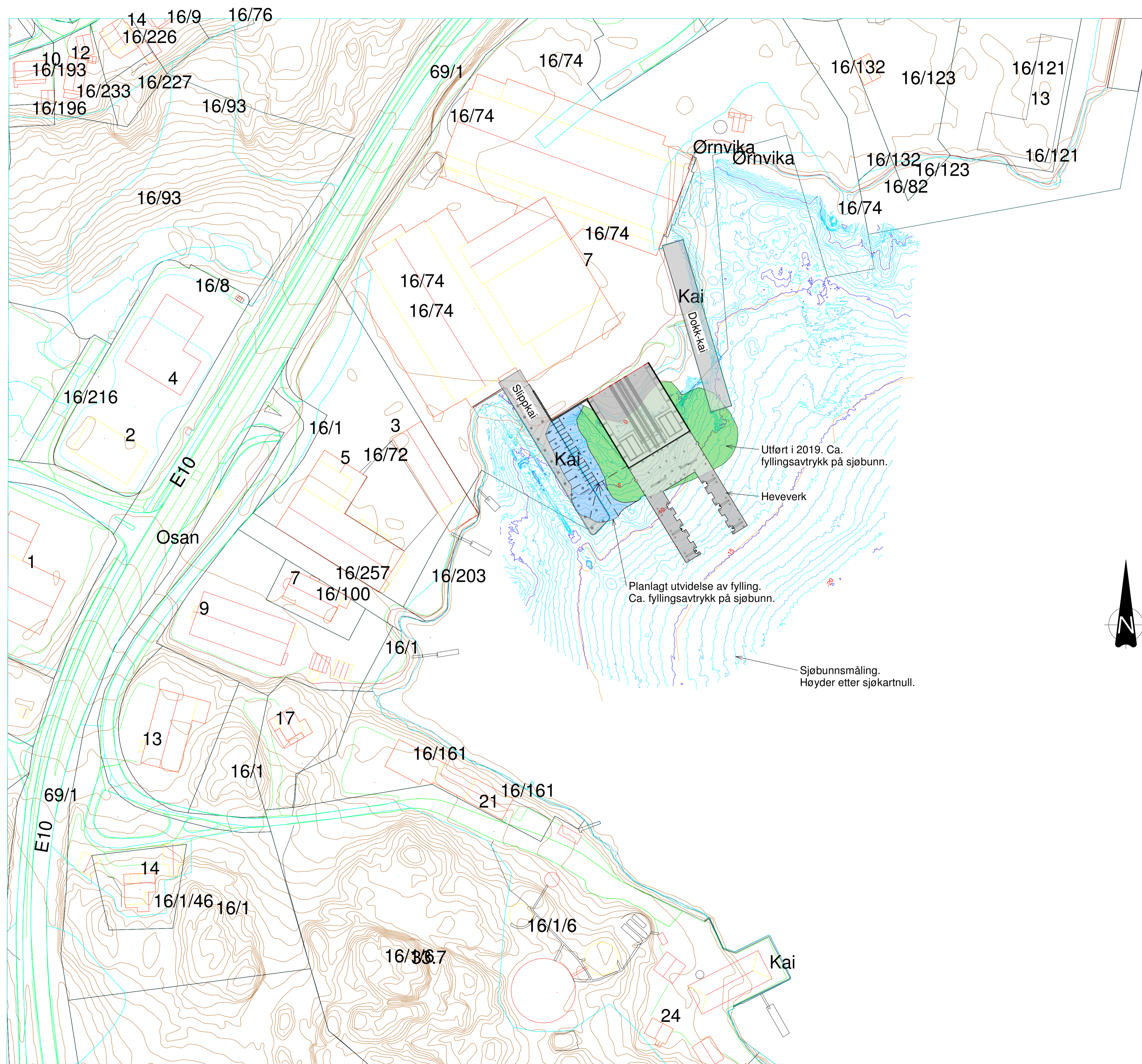
Plan - Fyllingsavtrykk sjøbunn 1 : 1000
