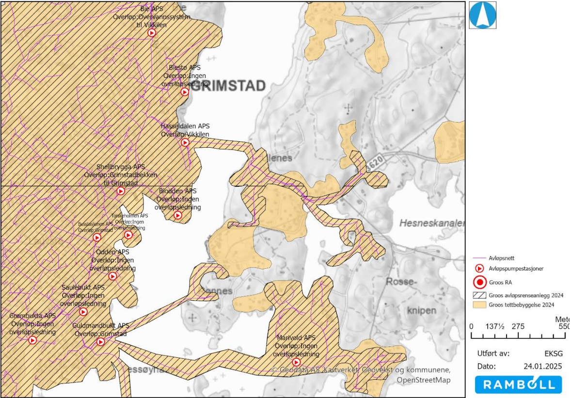
Figur 11 Overløpspunkter innenfor rensedistriktet
