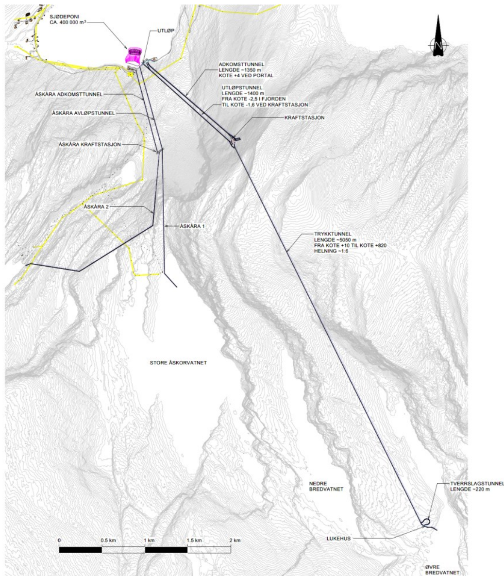
Figur 2 Kartskisse Bredvatn kraftverk (Kjelde: Norconsult, på oppdrag frå SFE)
